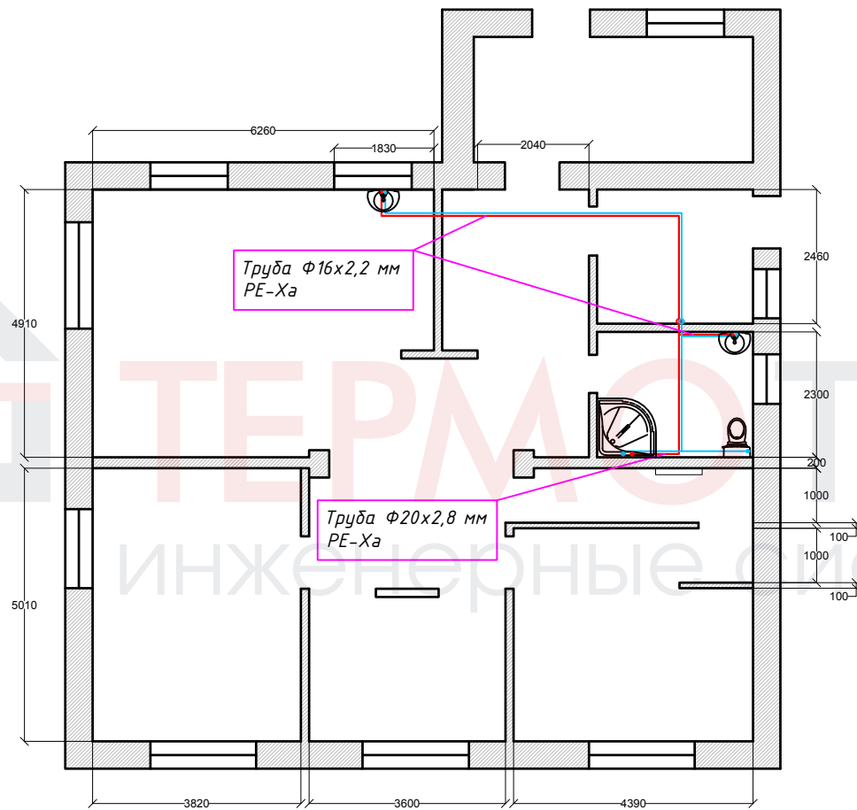
Рисунок 4 - Схема прокладки магистралей водоснабжения
