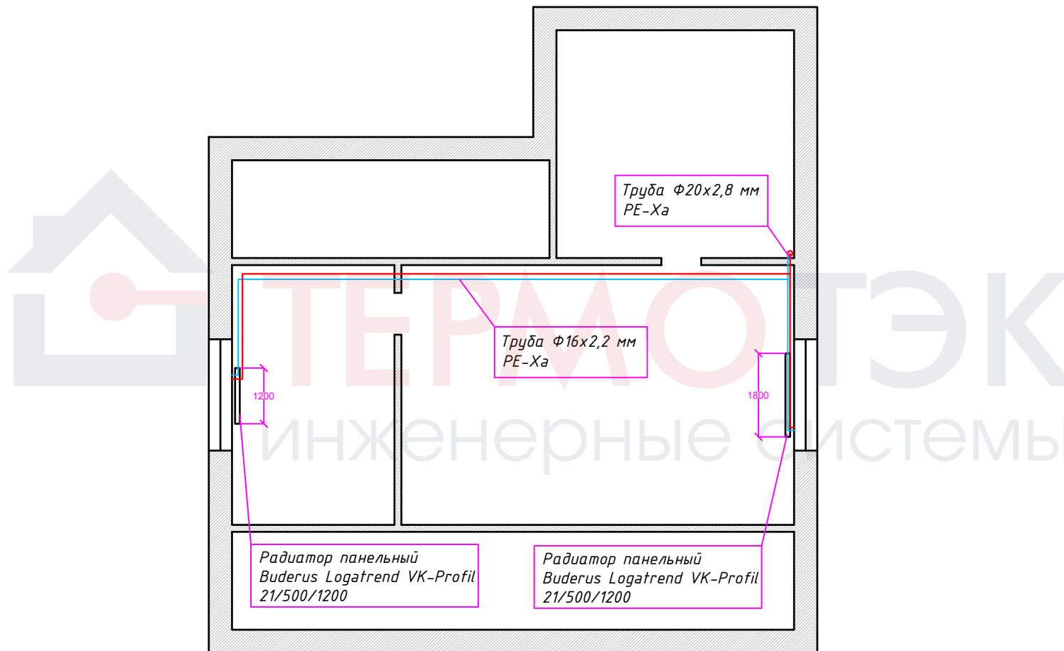
Рисунок 3 - Схема радиаторного отопления на 2 этаже
