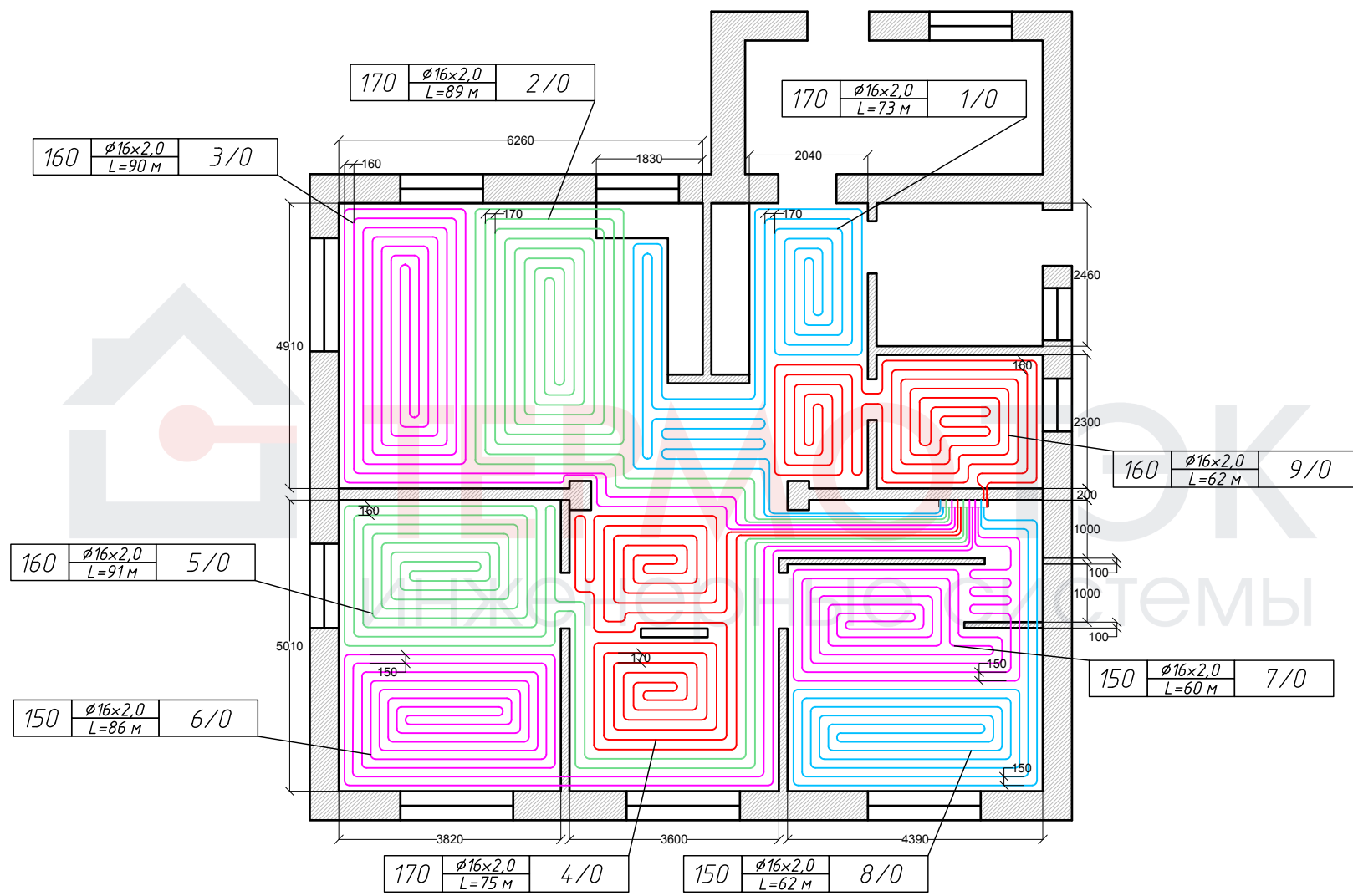
Рисунок 1 - Схема укладки трубы теплого пола на 1 этаже
