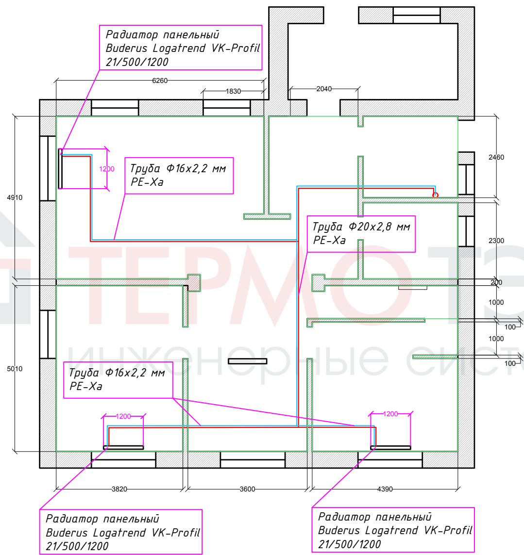
Рисунок 2 - Схема радиаторного отопления на 1 этаже
